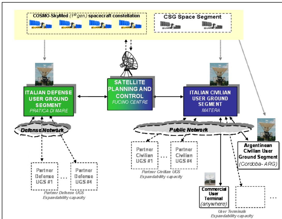
Figura 3 – Schema concettuale dell'architettura del sistema COSMO integrato (prima e seconda generazione)
