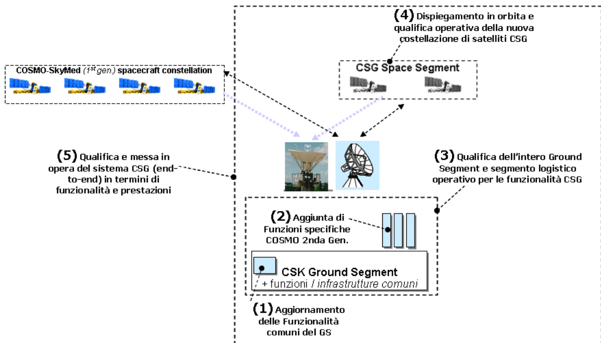
Figura 4 – Strategia di dispiegamento delle funzionalità e degli elementi del sistema COSMO di Seconda Gen.
